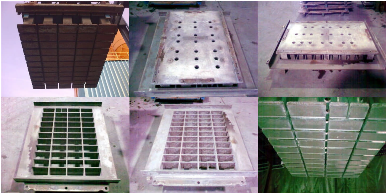
06. Rechteck 20 x 10 x 8 cm 43 + 2- teilig mit Fase.
